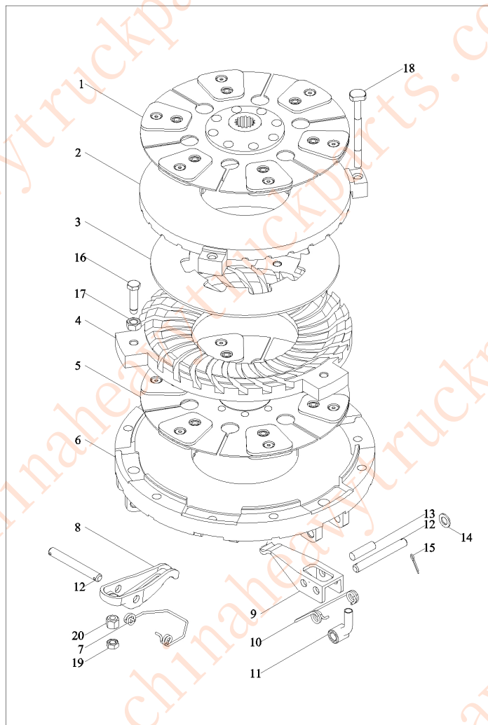
TB550.211A 离合器分总成
