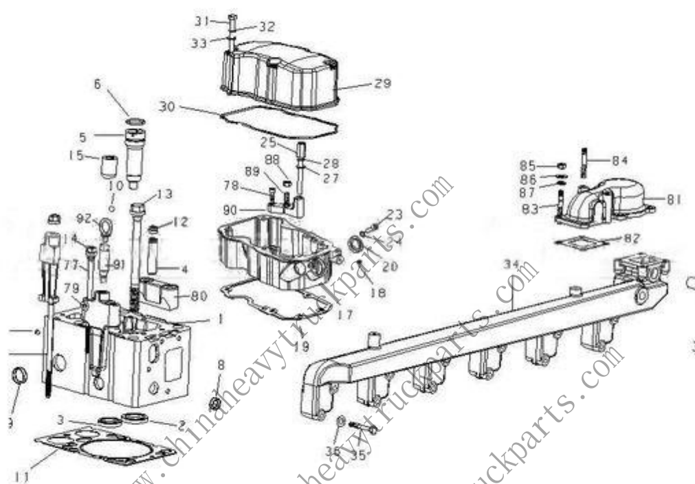
气缸盖和配气机构（四气门）
