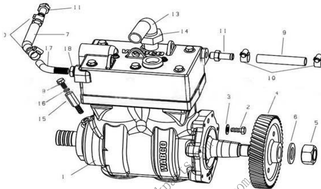
双缸水冷空压机
