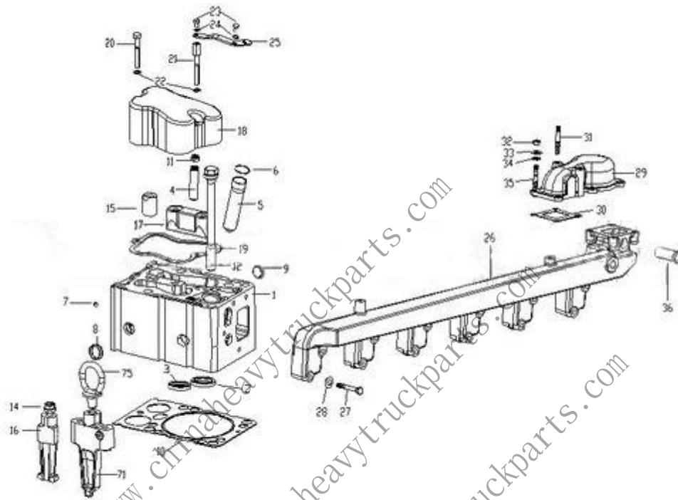
气缸盖和配气机构（两气门）
