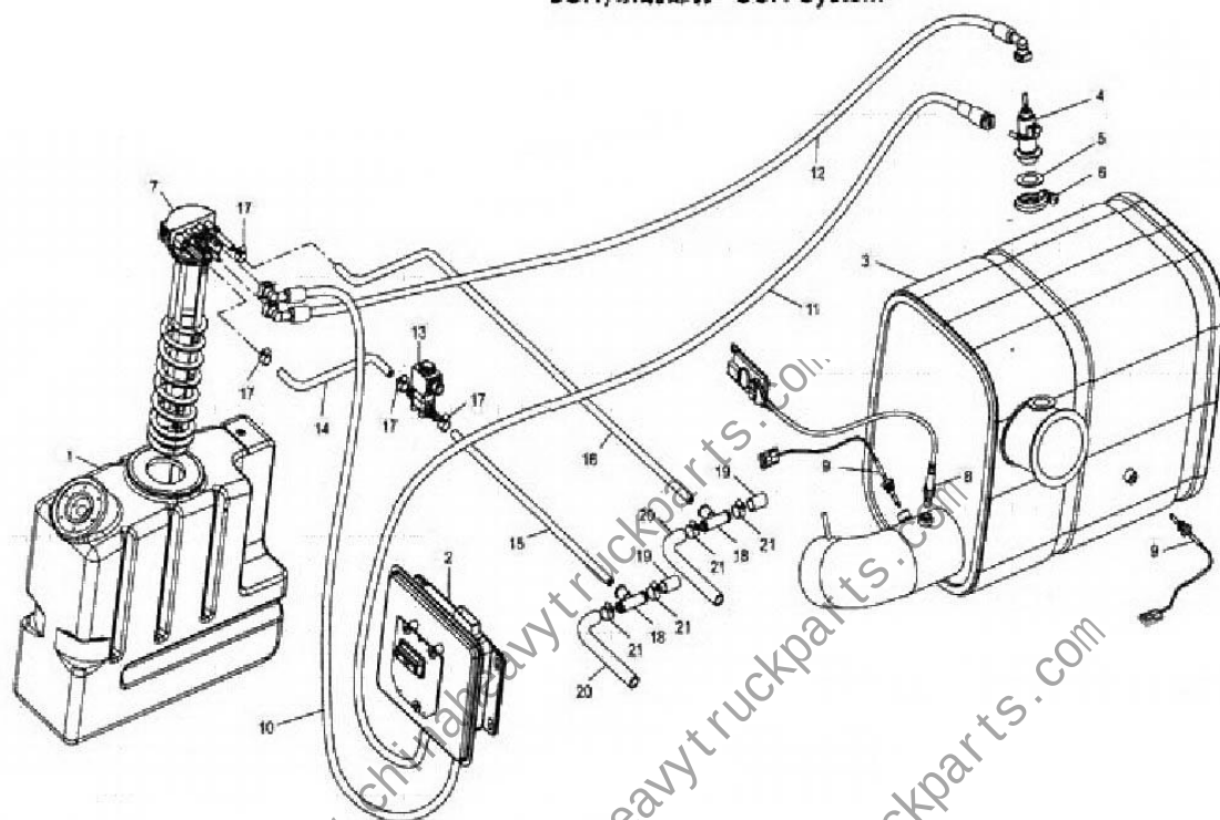
SCR)系统部分 SCR System
