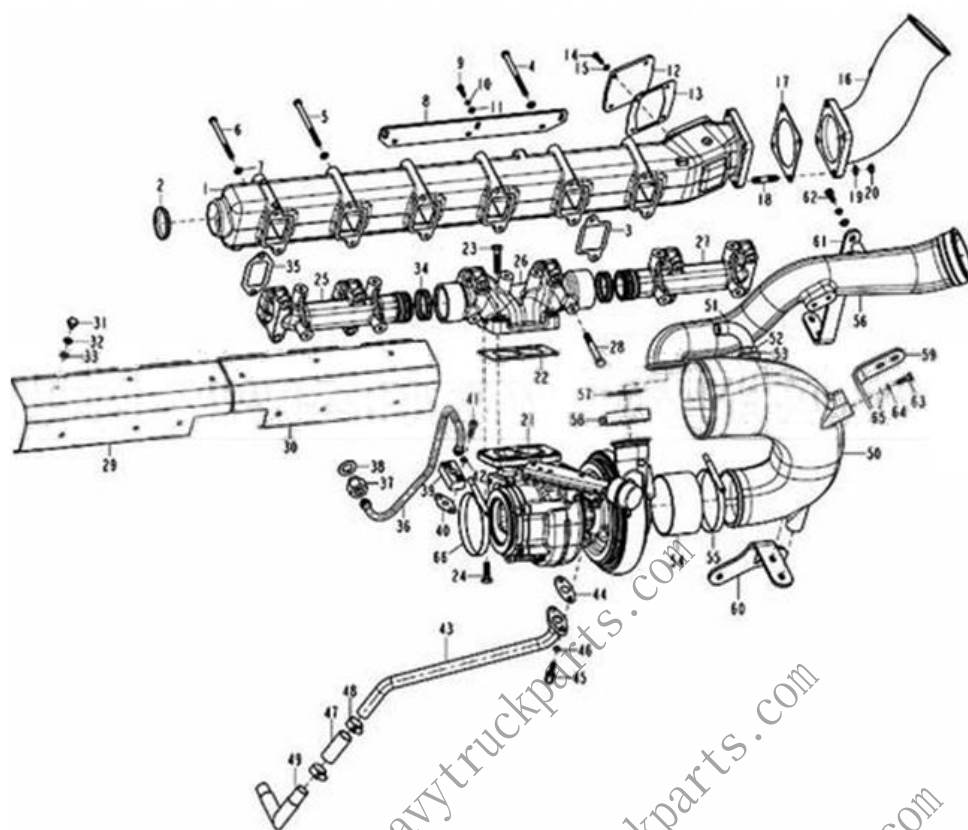
进排气系统
