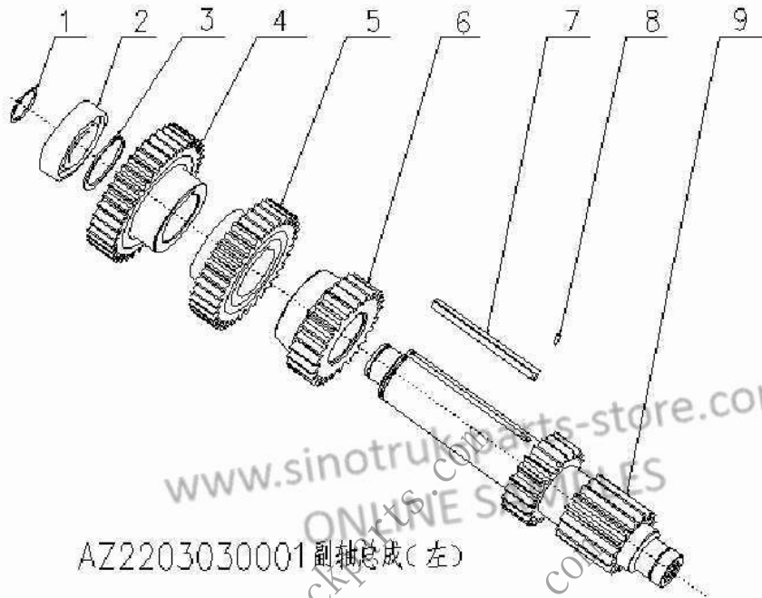
副轴总成（左）
