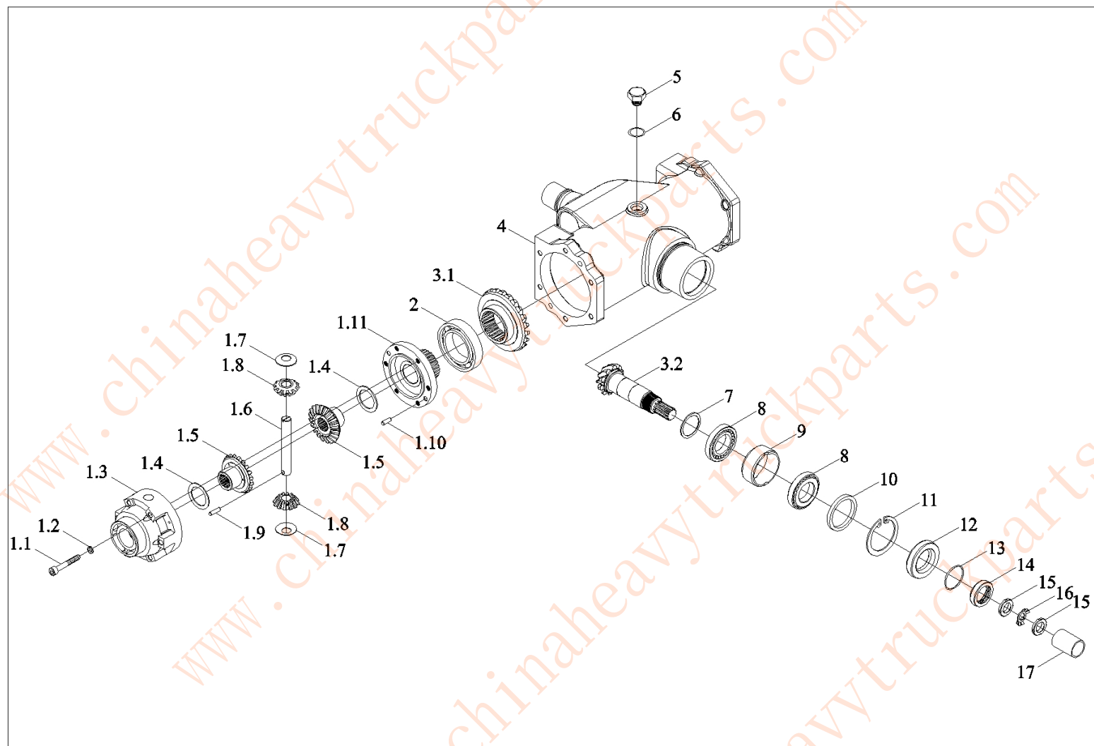
TC02311020000 前驱动桥总成-6
